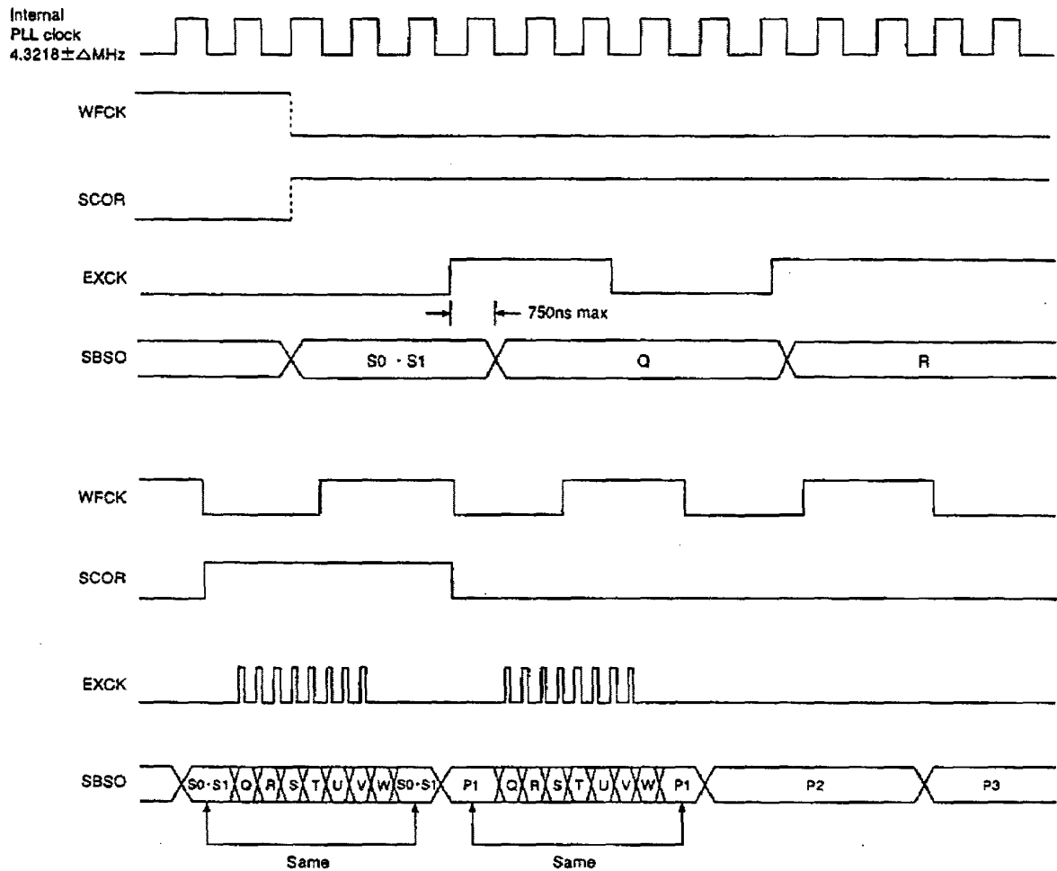
Subcode P.Q.R.S.T.U.V.W Read Timing
